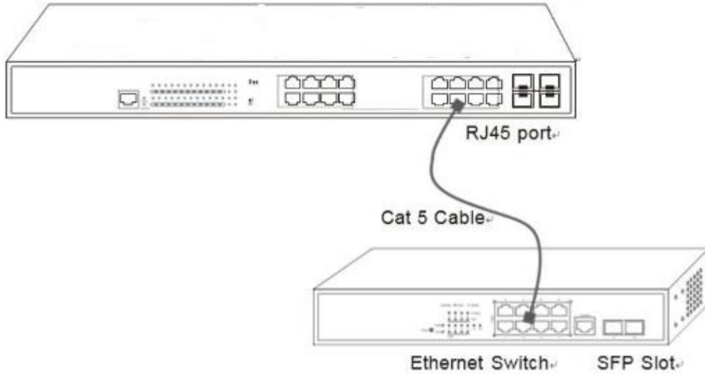
Şekil 3-8 Base-TX portunu ve diğer Ethernet terminallerini bağlama
