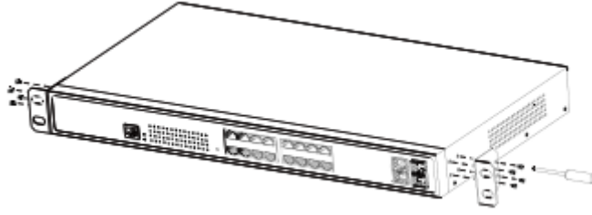
Şekil 3- 1 Anahtarın kutuya sabitleme
