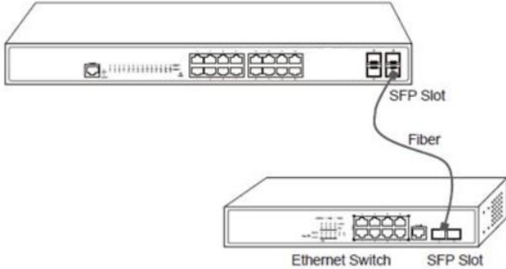
Şekil 3-6 SFP portunu ve diğer Ethernet terminallerini bağlama
